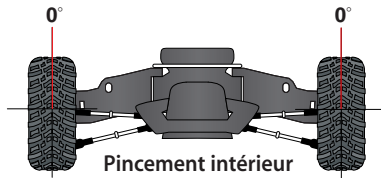
Pincement intérieur
