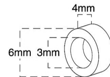
3x6x4mm Spacer
