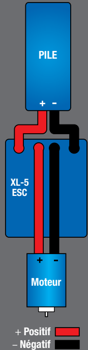
Diagramme de câblage du contrôleur XL-5
